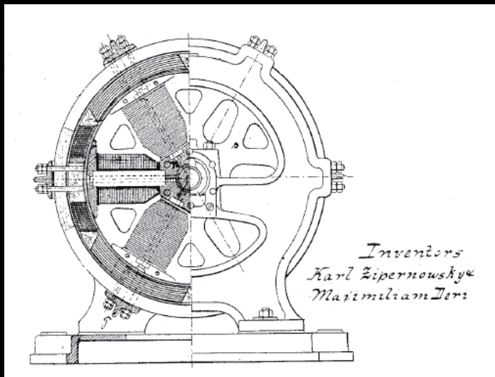
Динамо машина за производство на електрична енергија
